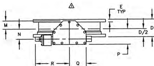
ACTUATOR POSITION 1
